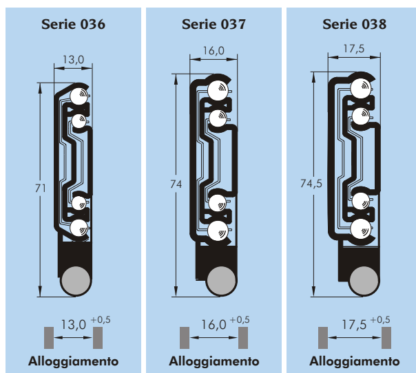
Guida ad estrazione totale Schöck con « Soft Control 2 » Montaggio consigliato con ammortizzatore verso il basso
