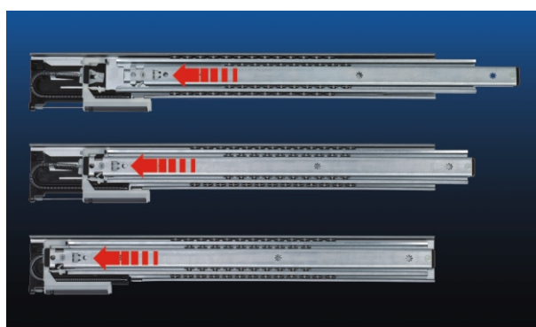
Guida ad estrazione totale Schöck con « Soft Control 2 » Montaggio consigliato con ammortizzatore verso il basso
